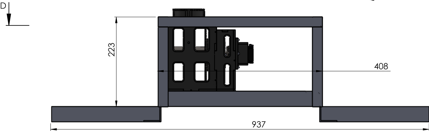
Vista perfil
