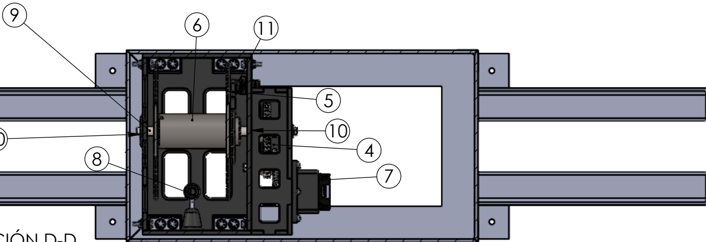
SECCIÓN D-D ESCALA 1:4.5
