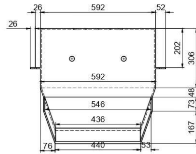
VISTA ELEVACIÓN ESC 1:20
