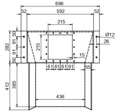
VISTA PLANTA ESC 1:20
