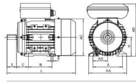
IM B3
