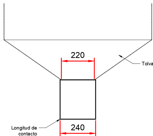
Esquema de longitud de contacto del cilindro
