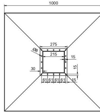
VISTA PLANTA ESC 1:20
