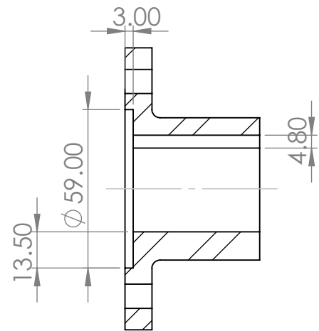
SECCIÓN P-P
