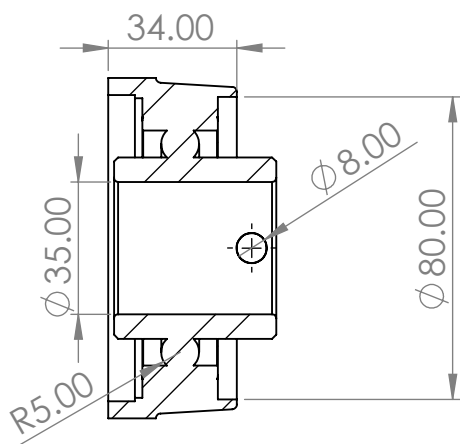
SECCIÓN D-D
