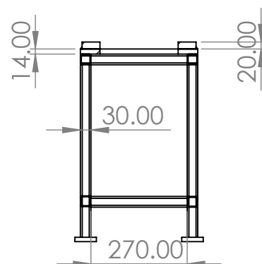
SECCIÓN A-A ESCALA 1 : 15
