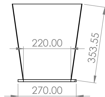
SECCIÓN N-N ESCALA 1 : 10
