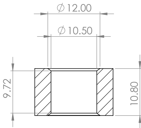
SECCIÓN S-S
