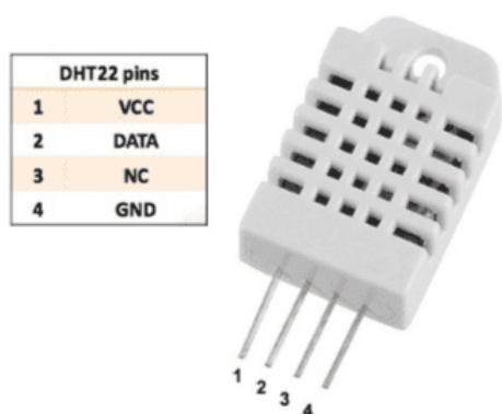
Figura 19 Sensor de temperatura
