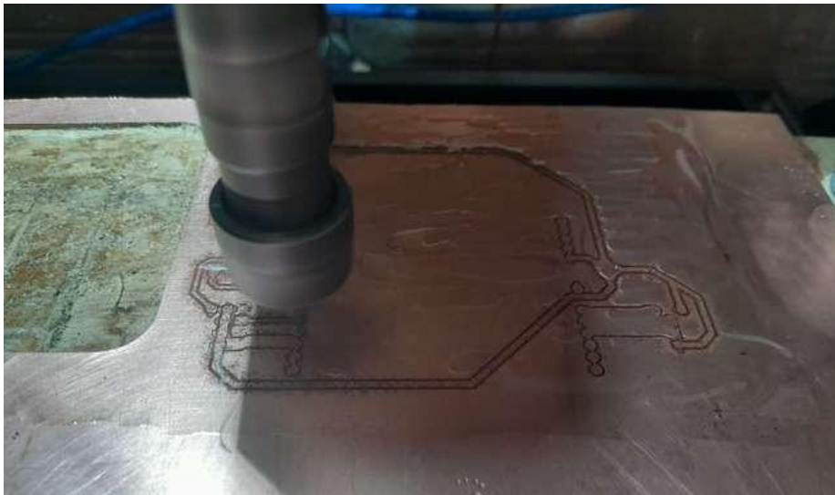
Figura 35 Elaboración de PCB
