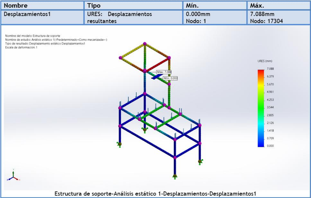
Figura 11 Análisis de desplazamientos
