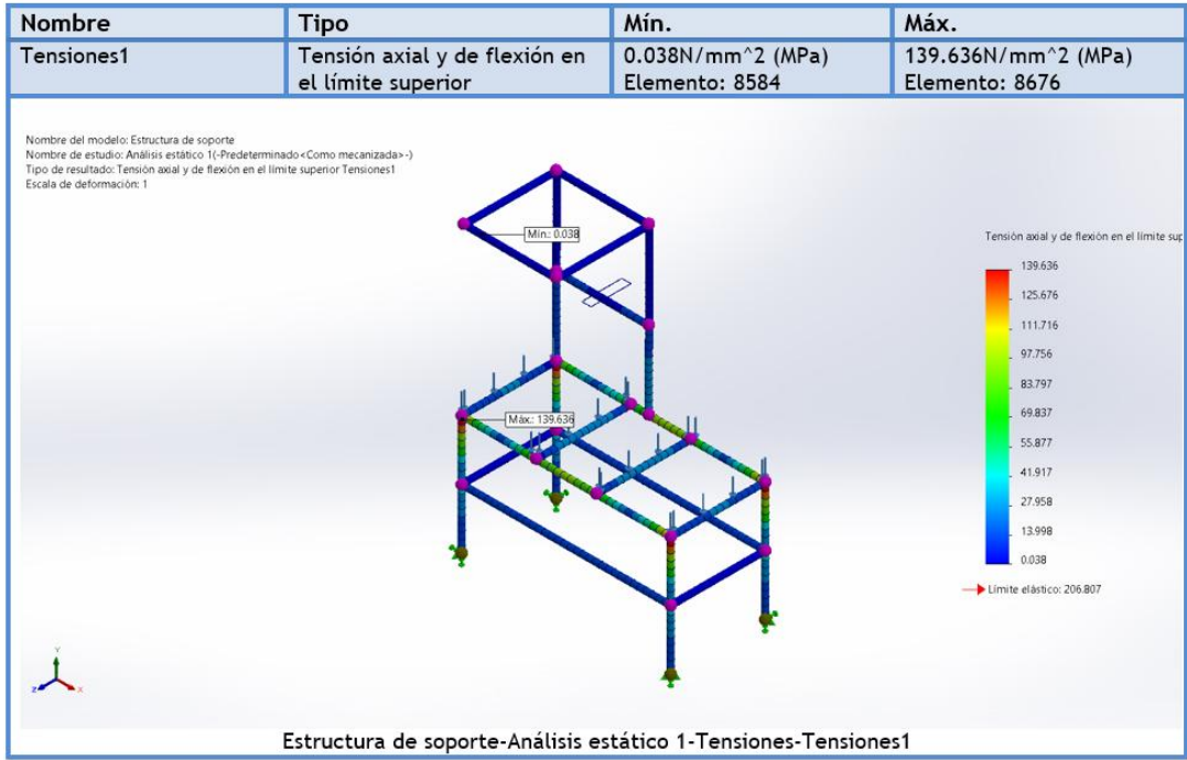
Figura 10 Análisis de tensiones
